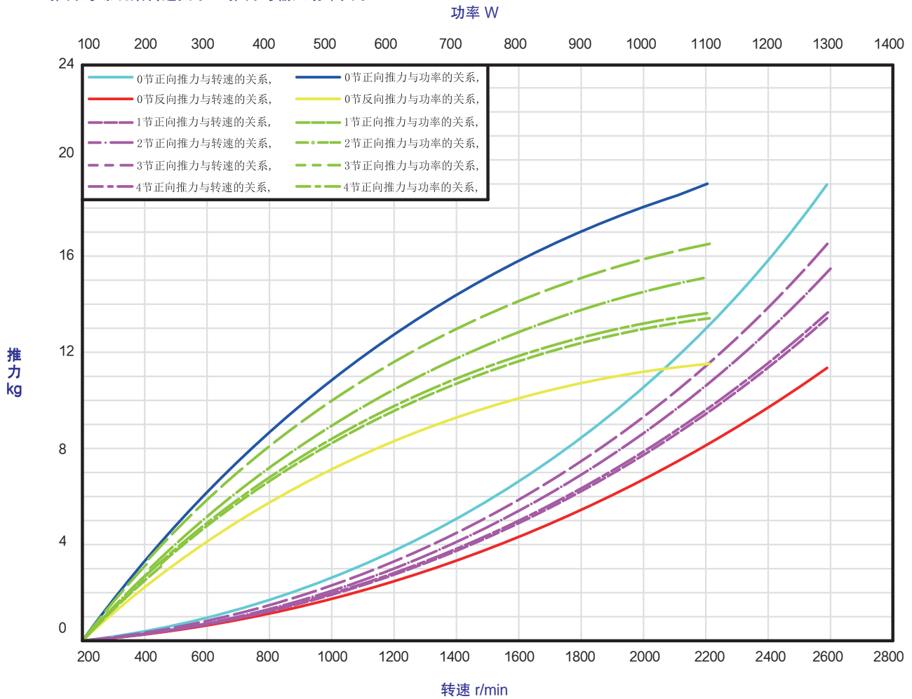
推力与螺旋桨转速关系 &amp; 推力与输入功率关系
